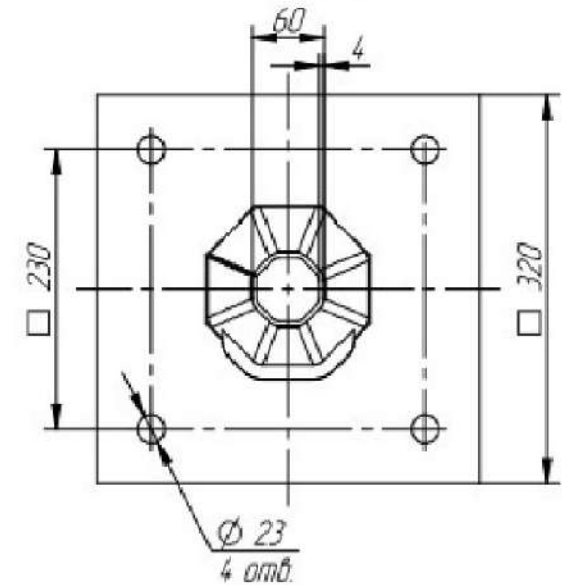
Вид сверху
