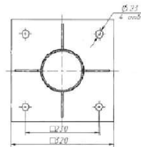
Вид сверху
