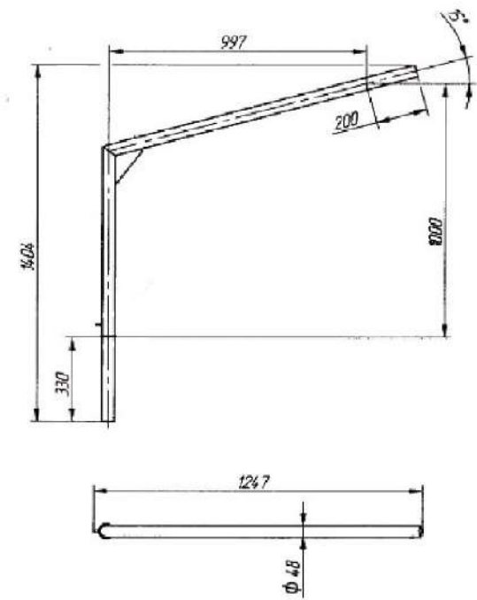
Кронштейн
