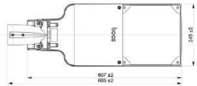
Светильник
