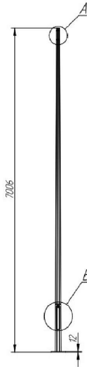
Опора
